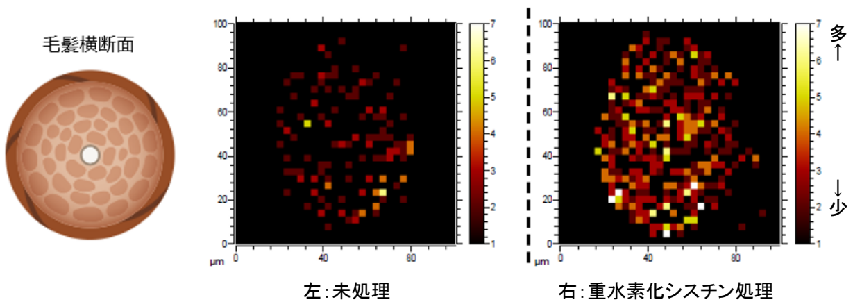
図1 ヘアカラー製剤に配合したシスチンの毛髪への浸透性観察(TOF-SIMS 測定※3)
