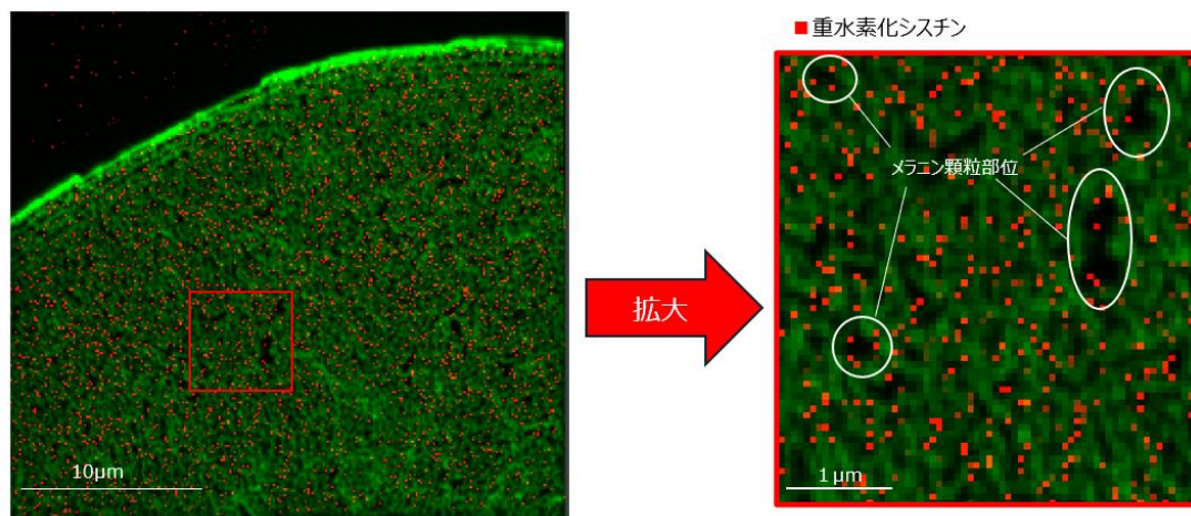
図2 ヘアカラー製剤に配合したシスチンの毛髪浸透部位(Nano-SIMS 測定※4)
